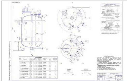
Аппарат вертикальный с эллиптическими днищами ВЭЭ1-1-2-0.6
