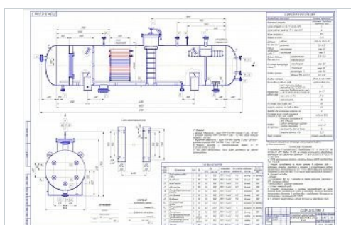
Нефтегазосепаратор НГС-II-0.6-1600-П-И
